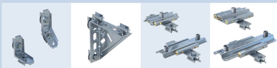
Conector angular CN CC 41 Stabil Escuadra de montaje WK CC Patín GS CC - H3G-PL Patín GS CC - 2G-PL
