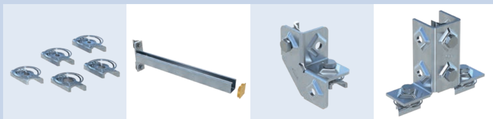
Tuerca soporte NT CC 41 Consola de montaje AK CC Conector angular EV CC 41-1 Conector angular EV CC 41-2
